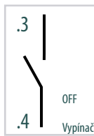
Označenie svoriek a funkcia univerzálného vysokovýkonného pomocného spínača Kontakt NO
