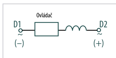
Označenie svoriek podpäťových spínačov
