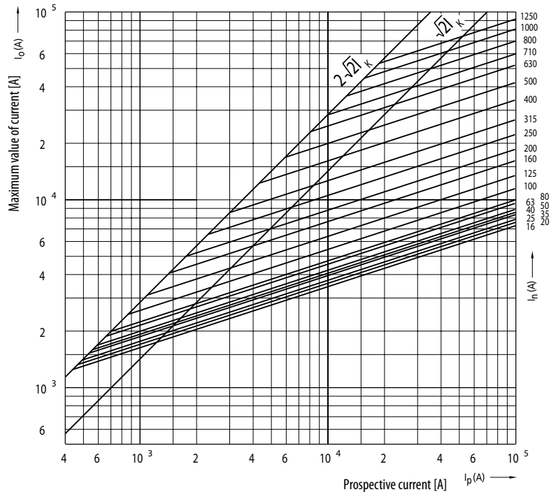
Skratová charakteristika
