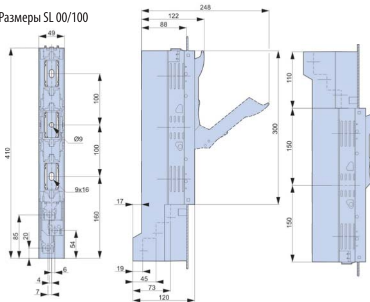
Размеры SL 00/185
