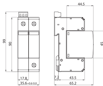
ETITEC C 1+1; 2+0
