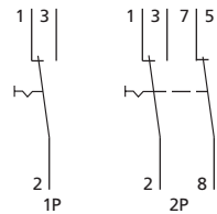
Wechselschalter
