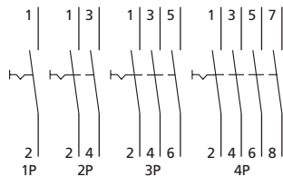
Schalter
