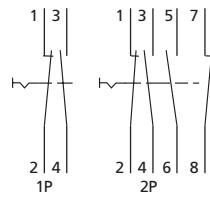
Steuerschalter
