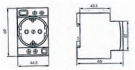
DIN Steckdose
