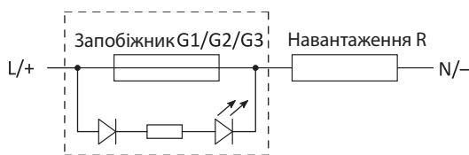
Внутрішня схема кола захисту
