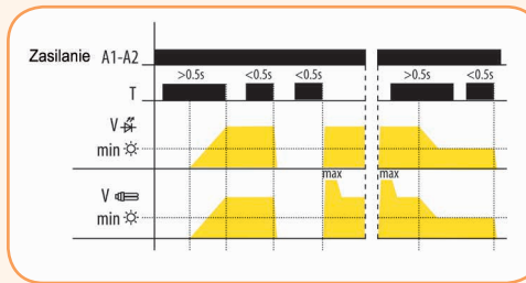
Diagram działania DIM-15
