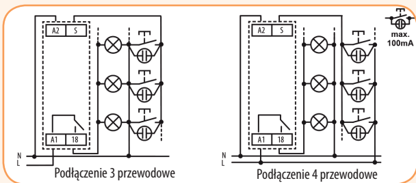
Układ podłączenia DIM-2
