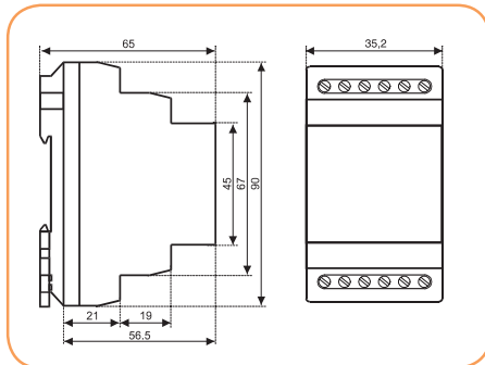
Automat zmierzchowy ETS-10b, ETS-16b
