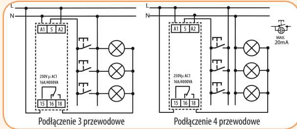
Układy podłączenia CRM-42
