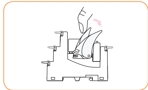
Sposób wyjmowania przełącznika z gniazdzka przy pomocy obejmy wyrzutnikowej
