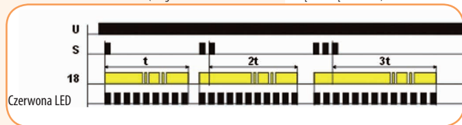
Diagram programowania CRM-42 (Długość świecenia można ustawić ilością naciśnięć klawisza)
