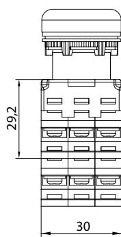
Napęd przycisku z 4 łącznikami i wspornikiem ze źródłem światła LED
