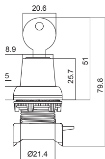
Napęd pokrętny kluczem
