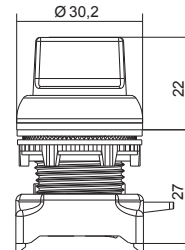
Napęd pokrętny piórkem
