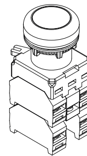
Napęd przycisku z 4 łącznikami i wspornikiem ze źródłem światła LED
